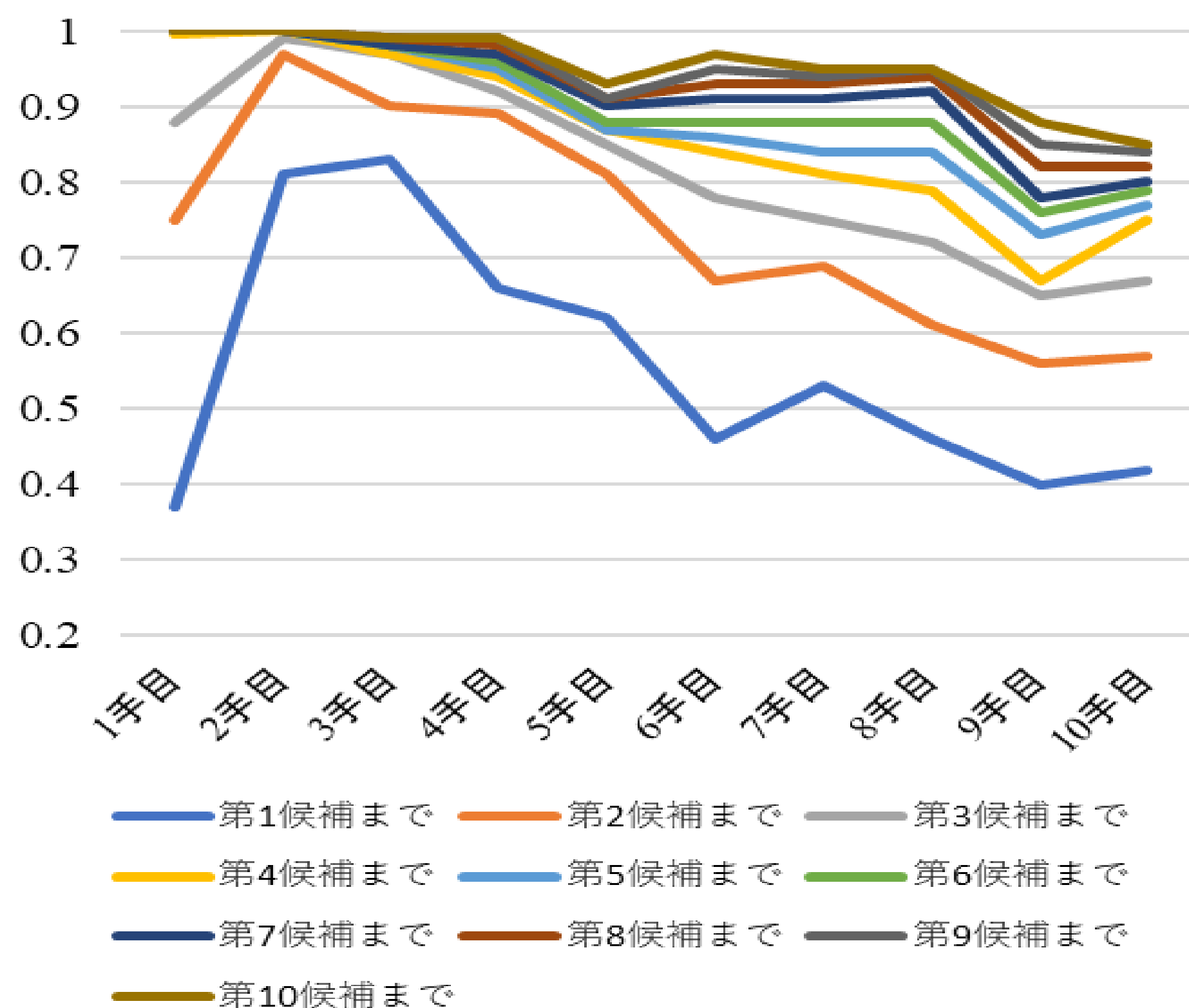
手数ごとの正解率
